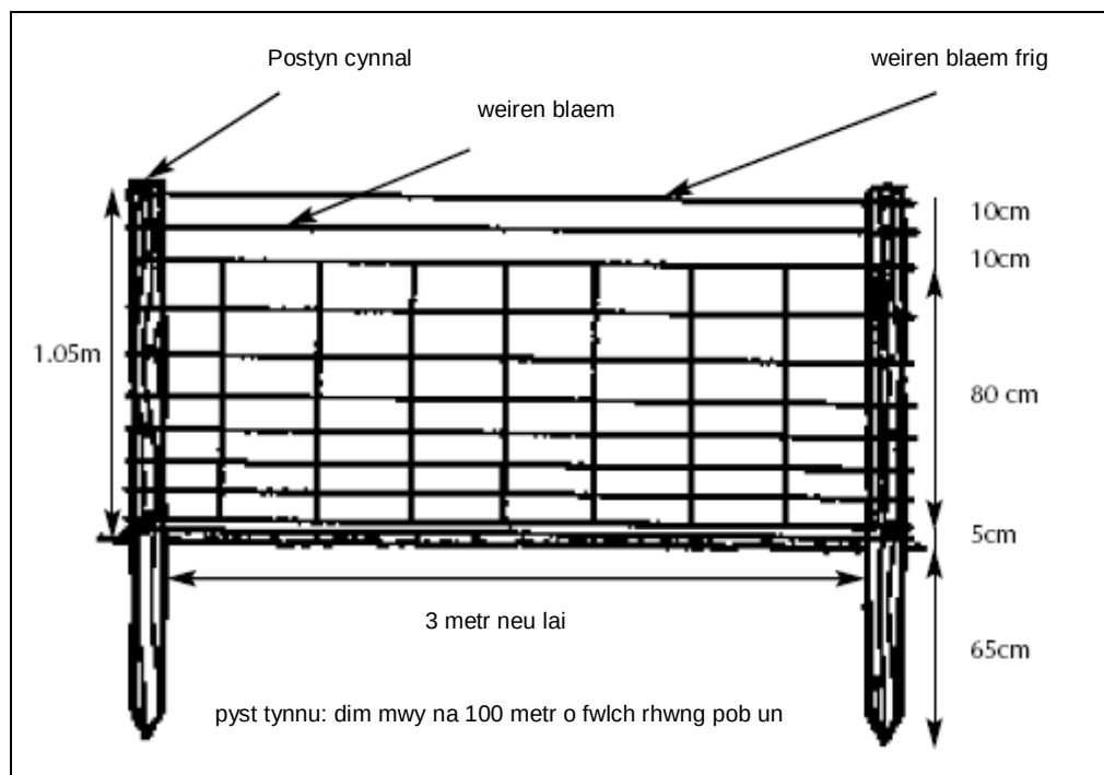
Diagram o ffensys netin ar gyfer stoc
