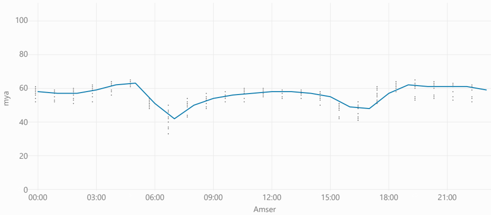
Proffil Cyflymder Traffig Fesul Awr: Tua'r Dwyrain
