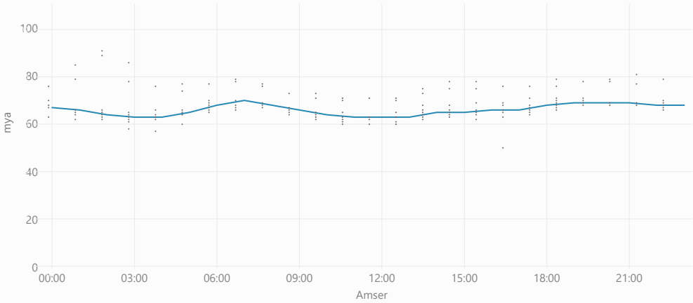
Proffil Cyflymder Traffig Fesul Awr: Tua'r Gorllewin
