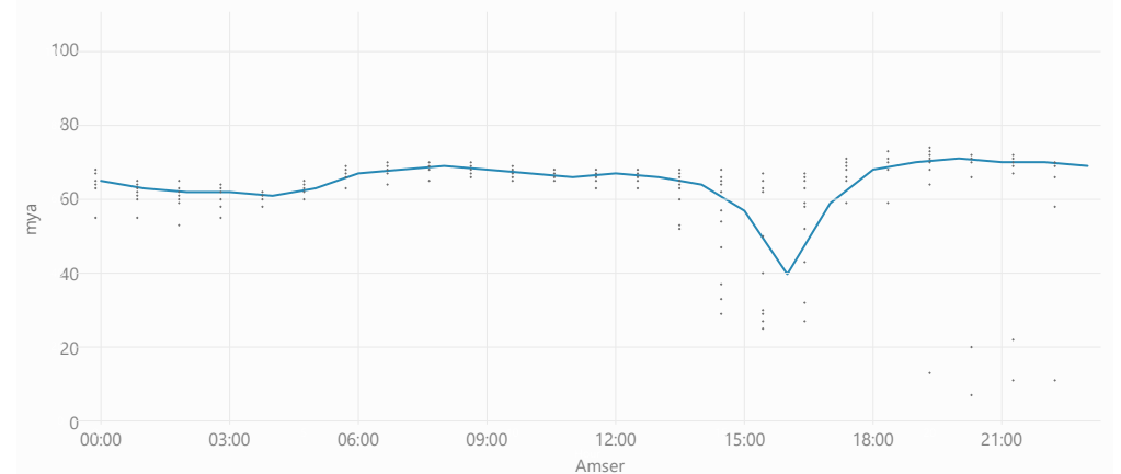
Proffil Cyflymder Traffig Fesul Awr: Tua'r Gorllewin
