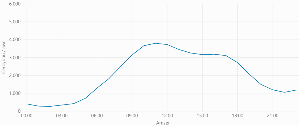
Proffil Llif Traffig Fesul Awr : Tua'r Dwyrain
