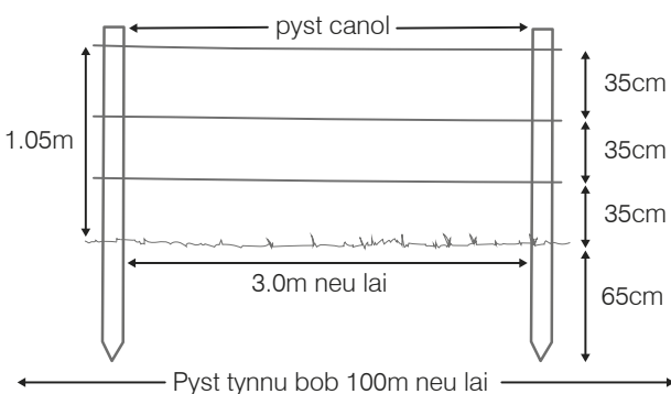
Diagram o Ffens Weiren Tri Llinyn
