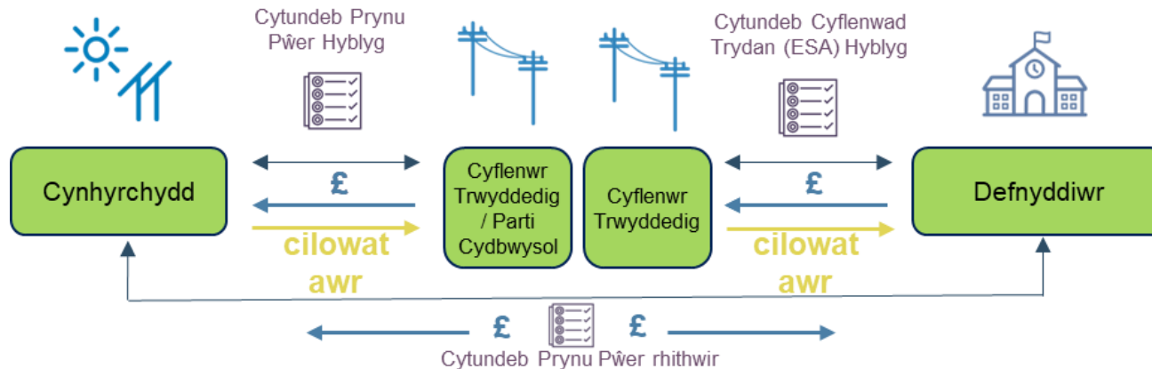
Ffigur 6: Diagram yn dangos Cytundeb Prynu Pŵer rhithwir / synthetig gyda defnyddiwr
