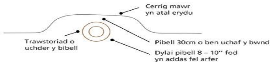
Gwlyptir mewn ffos (croestoriad o glawdd pridd)
