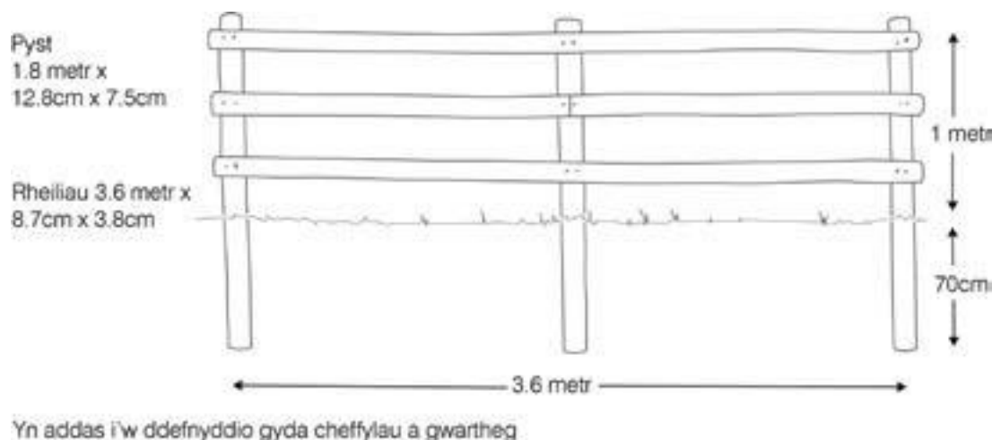
Ffens Postyn a Rheilen
